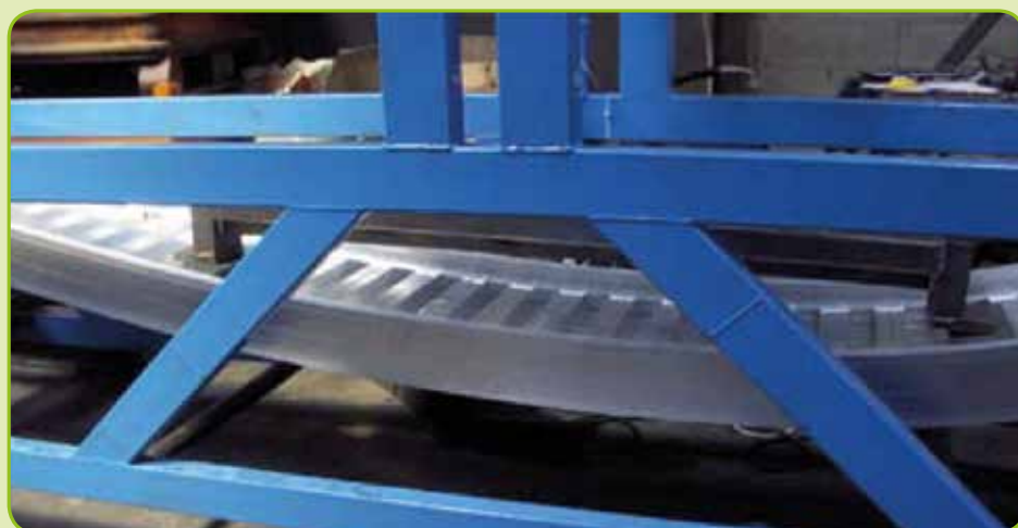
Rampa sottoposta a rottura.
